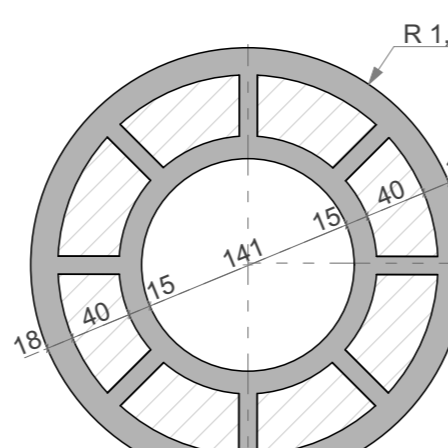
sez. A-A - quota 6,00
