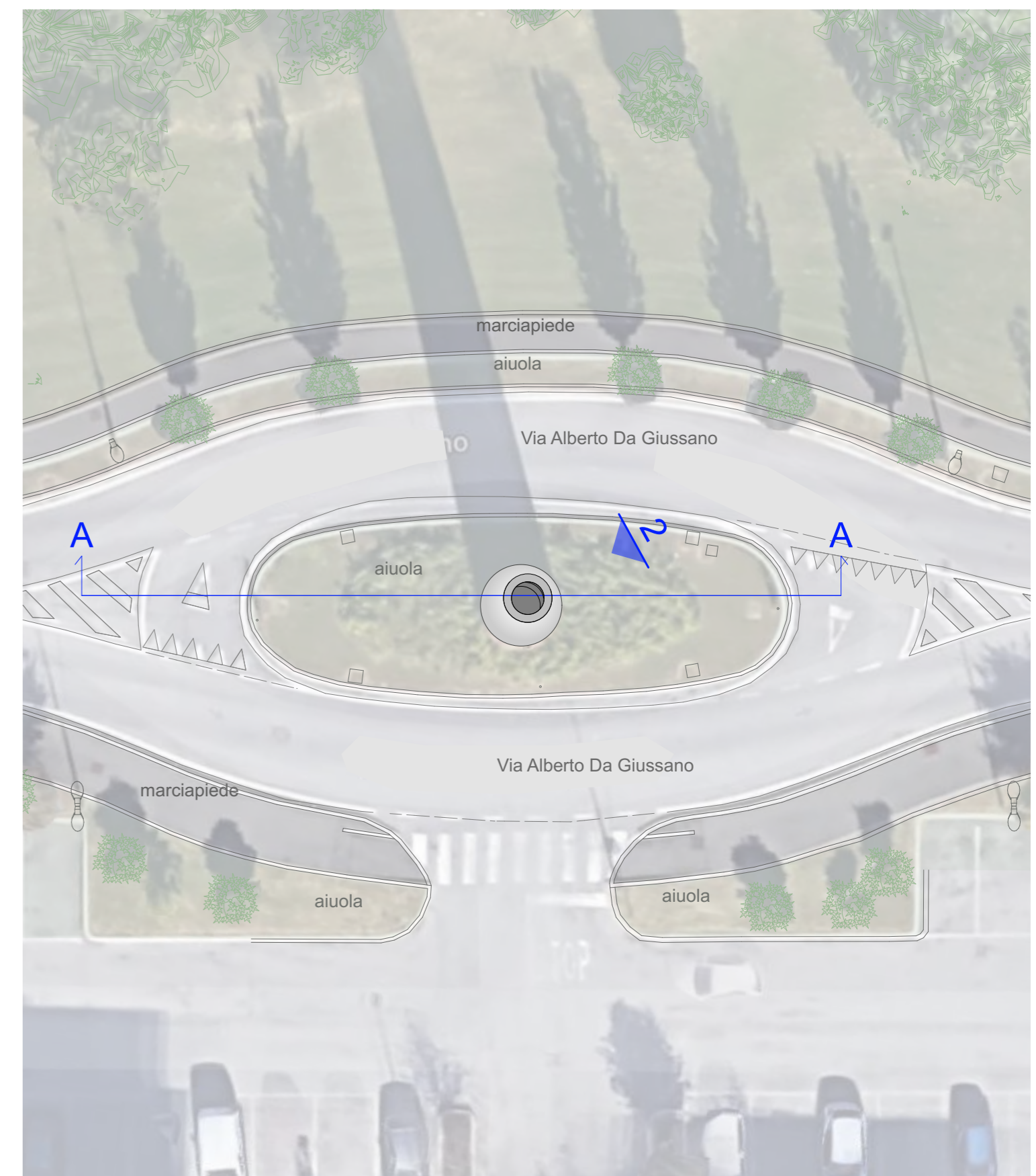
PLANIMETRIA 1:200
