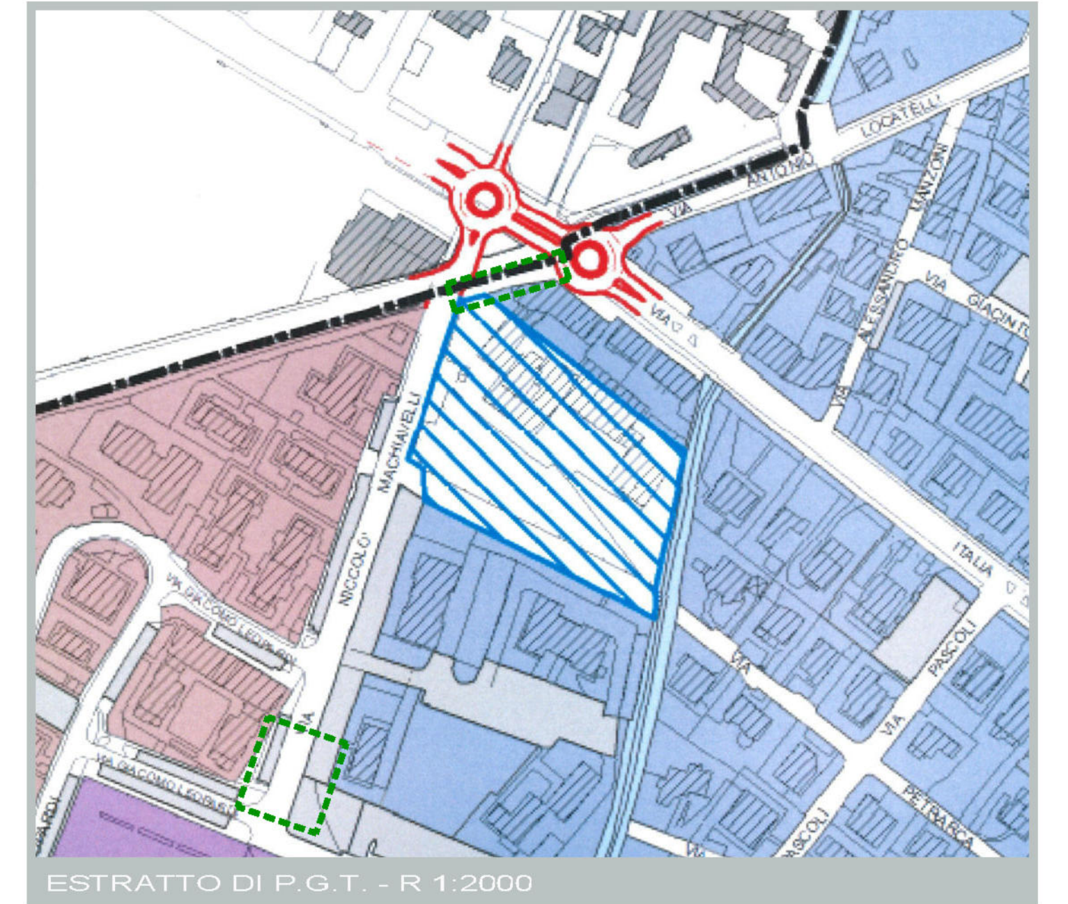
ESTRATTO DI P.G.T. - R 1:2000
