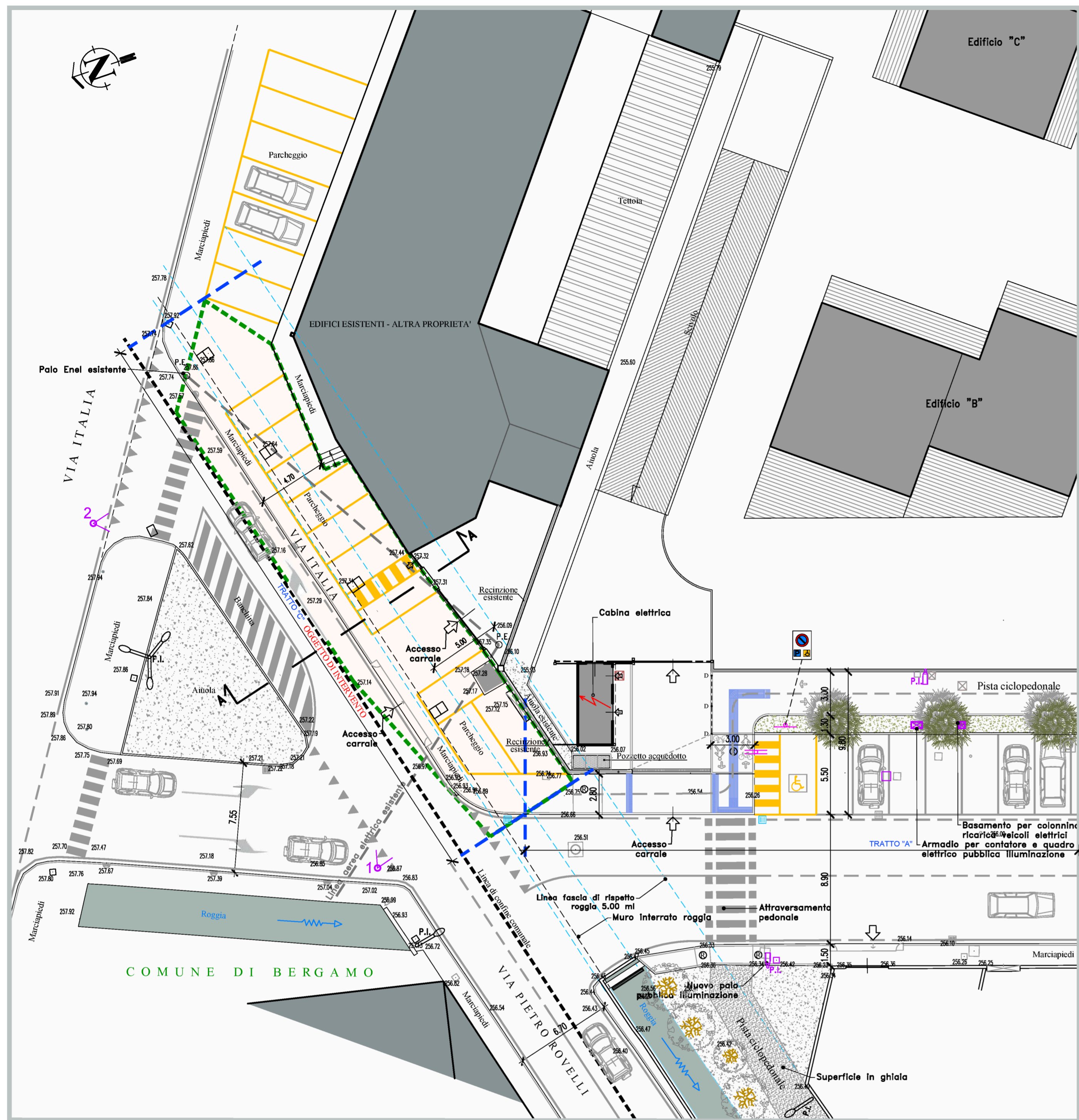
PLANIMETRIA GENERALE - TRATTO "C" [STATO DI FATTO] - R 1:200
