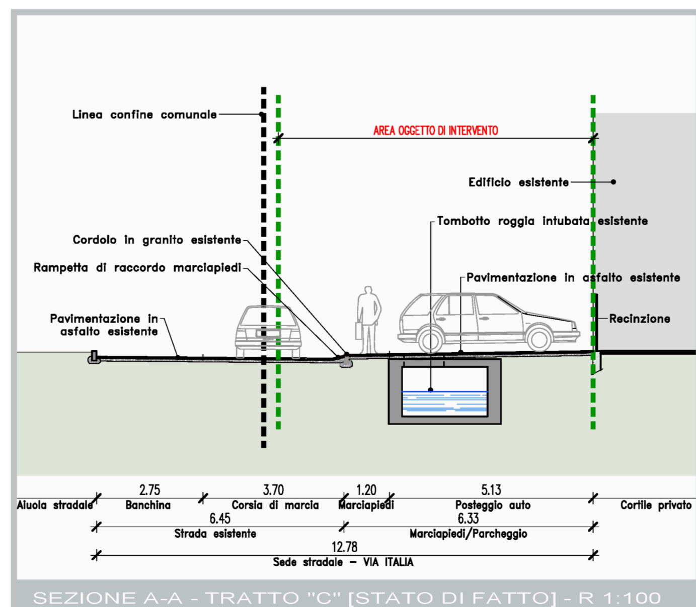
SEZIONE A-A - TRATTO "C" [STATO DI FATTO] - R 1:100
