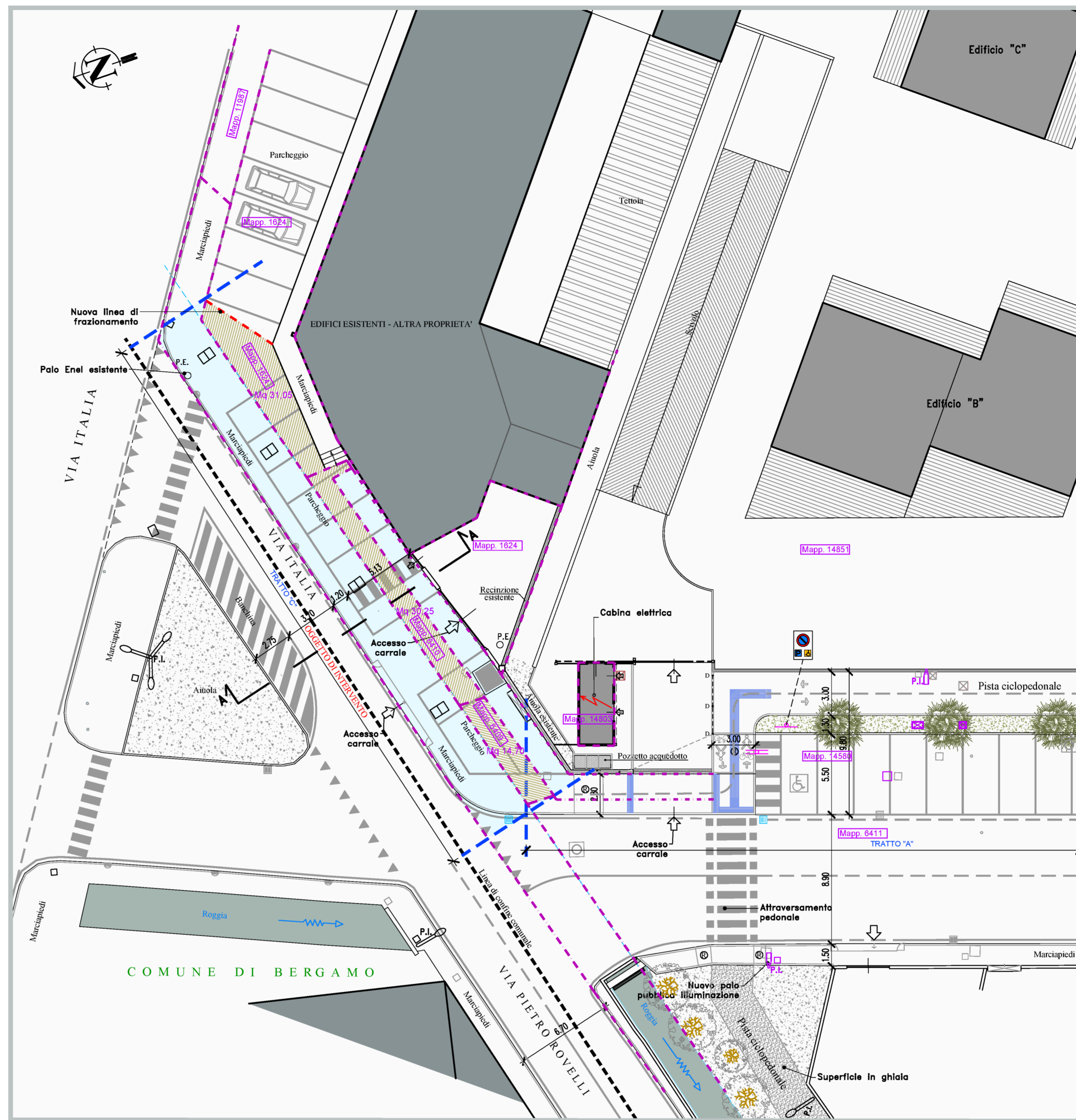
PLANIMETRIA GENERALE - TRATTO "C" [INDIVIDUAZIONE DELLE PROPRIETA'] - R 1:200
