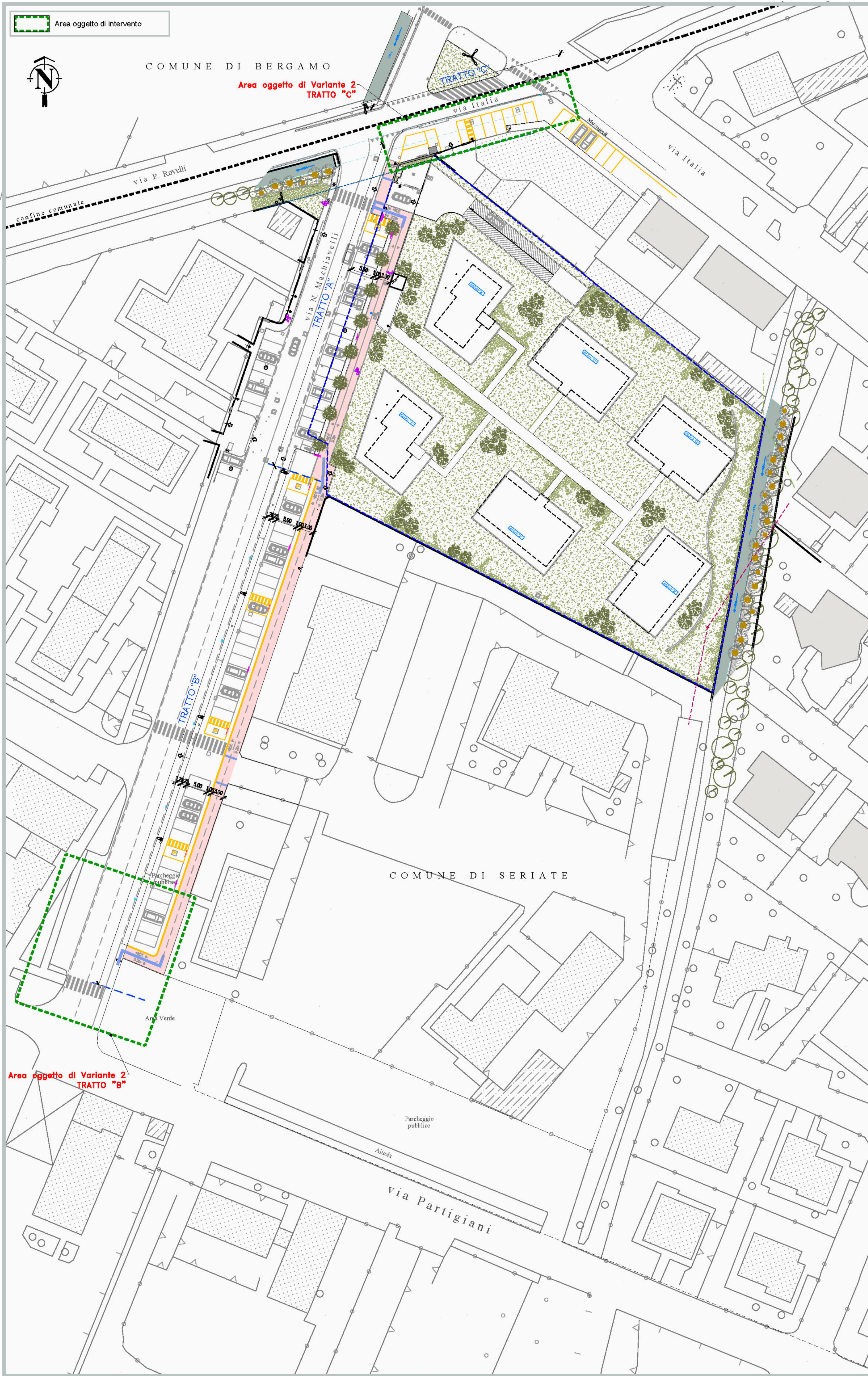
PLANIMETRIA GENERALE [STATO DI FATTO] - R 1:500
