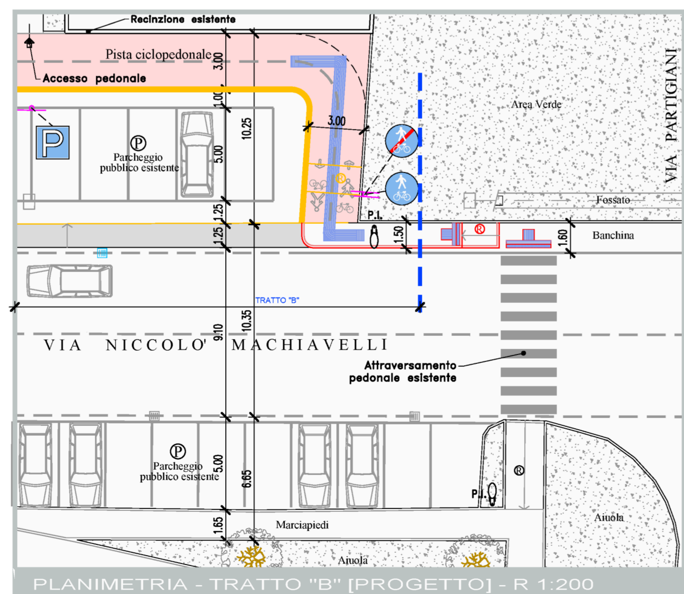
PLANIMETRIA - TRATTO "B" [PROGETTO] - R 1:200
