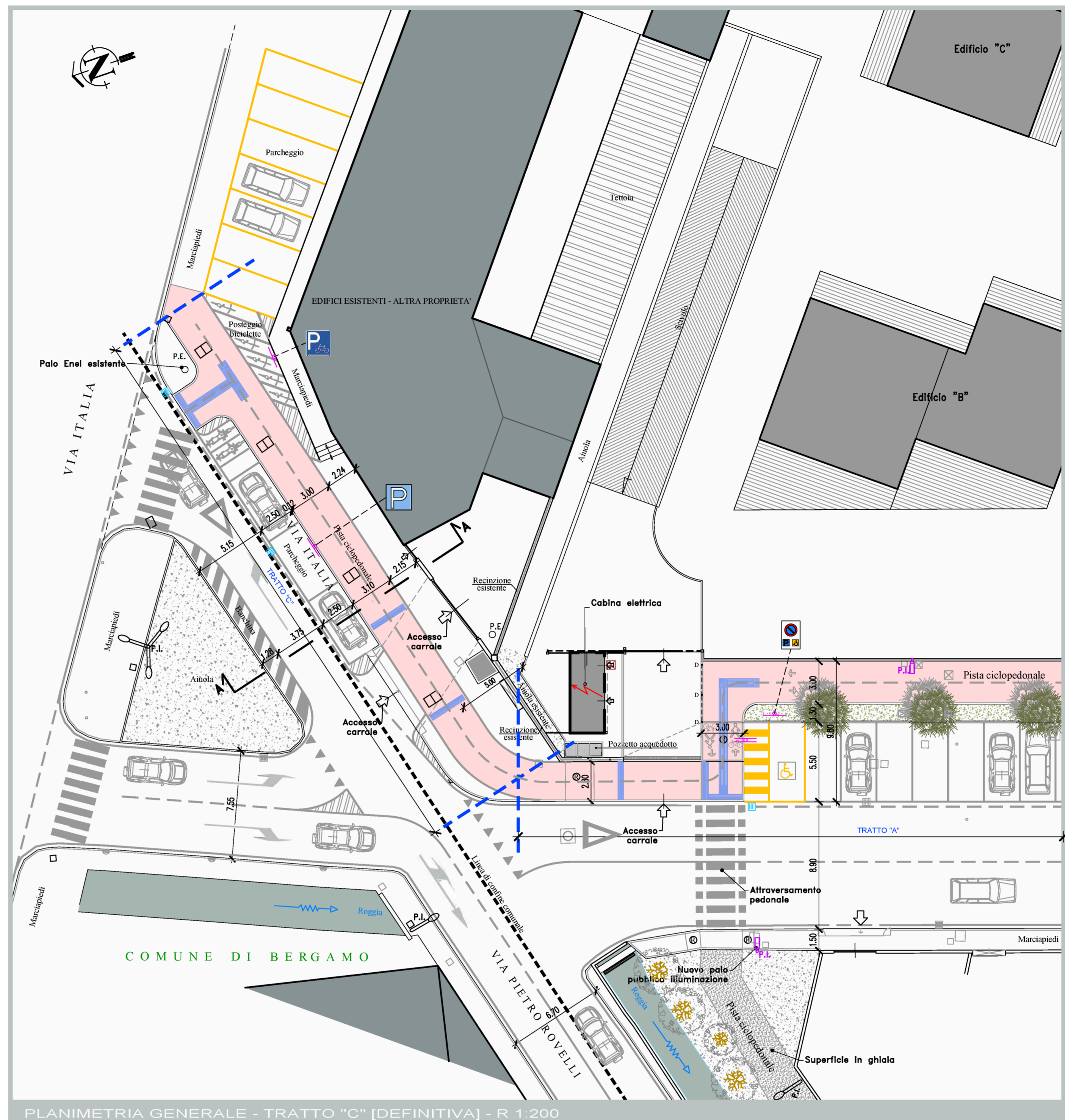
PLANIMETRIA GENERALE - TRATTO "C" [DEFINITIVA] - R 1:200
