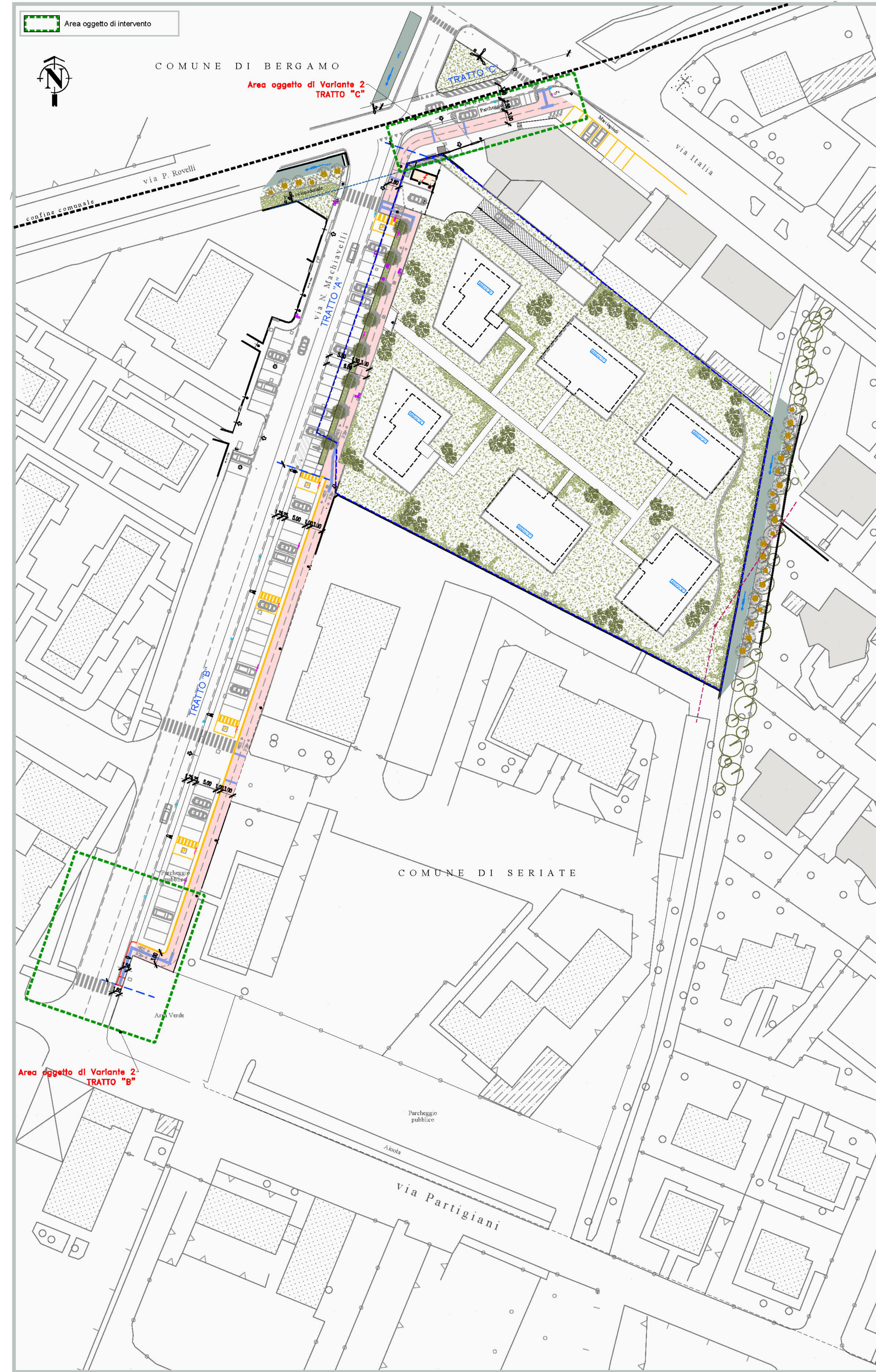
PLANIMETRIA GENERALE [PROPOSTA PROGETTUALE] - R 1:500
