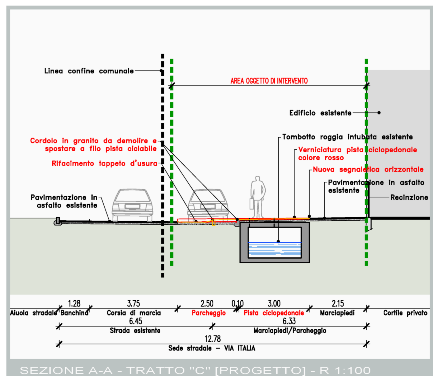
SEZIONE A-A - TRATTO "C" [PROGETTO] - R 1:100
