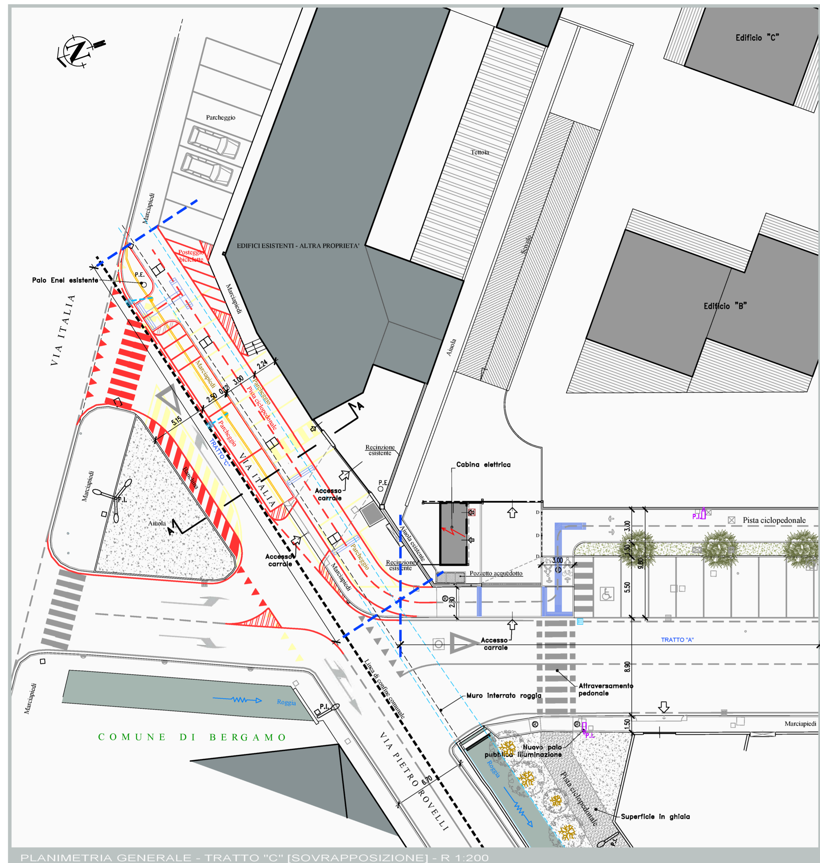
PLANIMETRIA GENERALE - TRATTO "C" [SOVRAPPOSIZIONE] - R 1:200
