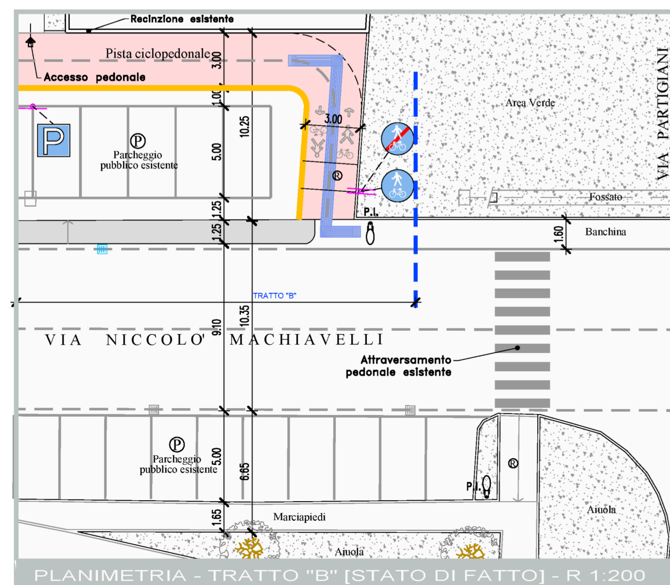
PLANIMETRIA - TRATTO "B" [STATO DI FATTO] - R 1:200
